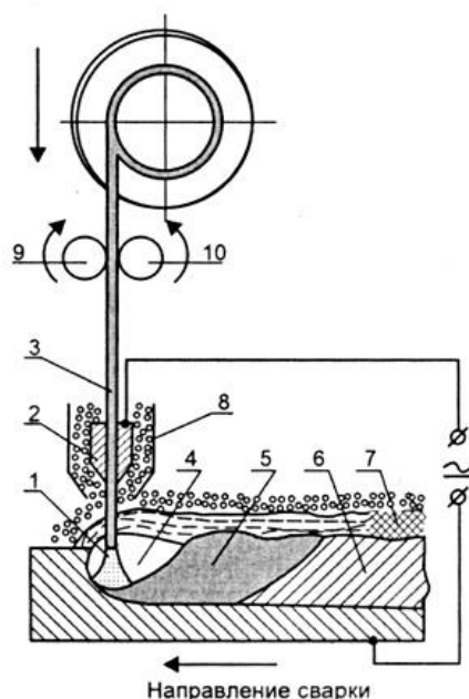
Схема процесса сварки под флюсом
