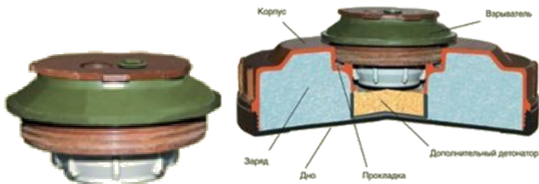
Внешний вид и устройство противотанковой мины
