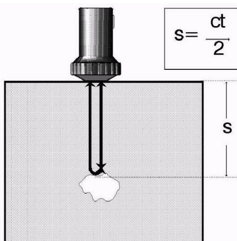
Принцип измерения времени и пути импульса
